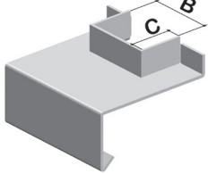
Pfeilerausschnitt mit Stehbord 3-seitig
