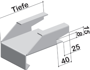
Spez. Klinkung Wetterschenkel KWS 40-25/8-15
