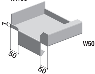
Wasserabweiser zu Steh- und Putzbord W7/50
