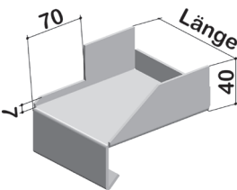
Stehbord St40-7/70
