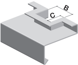
Pfeilerausschnitt mit Putzbord 3-seitig
