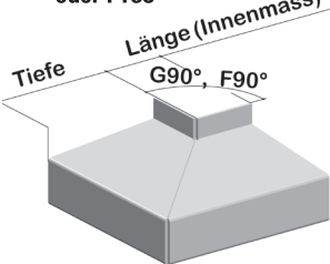
Gehrung mit Dilatation beliebige Winkel G90°, Formecke F90° oder F135°
