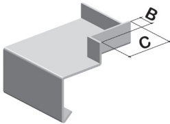
Pfeilerausschnitt mit Stehbord 2-seitig
